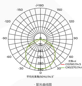
· 配光曲线图
